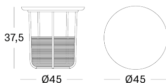
Vivi side table
